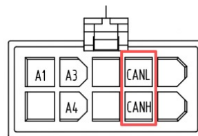
CAN节点D CONTROLLER
